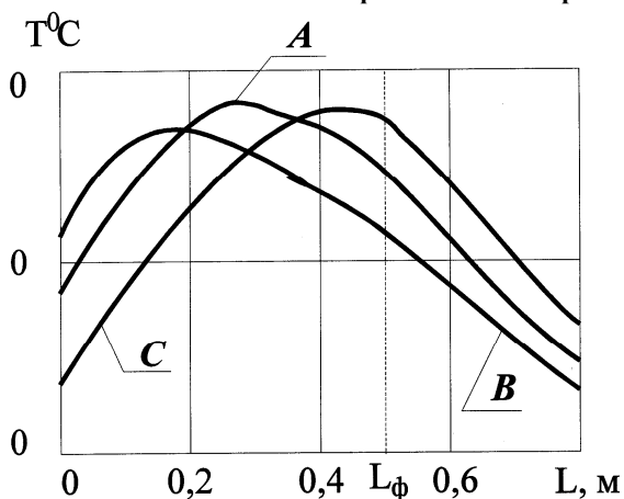
Рисунок 7 - Влияние расположения нагревателей по длине формирующего узла на изменение температуры в композите ( V_{\text{пр.}} - 0,4 м/мин; T_{\phi} - 220^{\circ}\text{C} )
