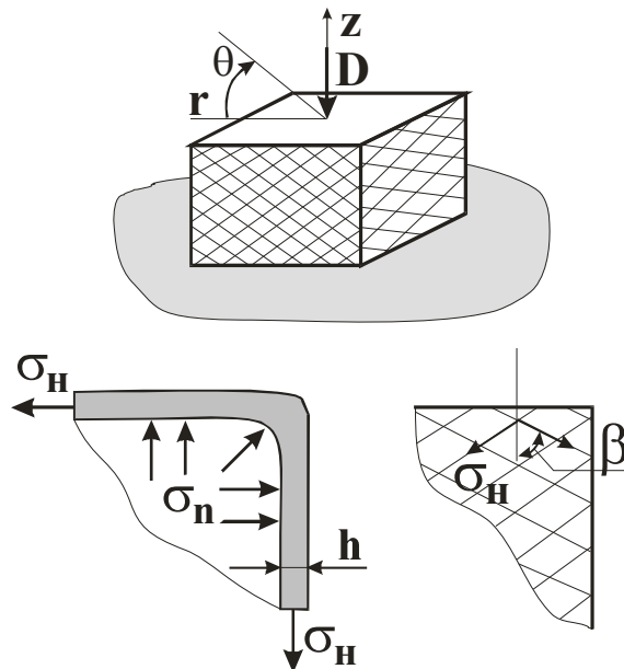
Рисунок 1 – К анализу напряженно-деформированного состояния при сжатии стержня с внешним слоем оплетки
