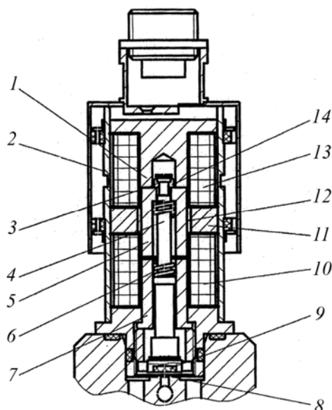
Рис. 1 – Конструктивная схема ЭМК с приводом типа ДТВ: 1 – верхний стоп; 2 – корпус клапана; 3 – шейка штока; 4 – шток; 5 – ползун (якорь); 6 – пружина; 7 – нижний стоп; 8 – седло; 9 – золотник с резиновой вставкой; 10 – нижняя обмотка; 11 – постоянный магнит; 12 – трубка разделительная; 13 – верхняя обмотка; 14 – шайба стопорная
