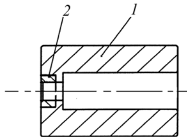
Рис. 10 – Ползун электромагнитного привода клапана с запрессованной втулкой: 1 – ползун (материал пруток 16Х); 2 – втулка (материал ХВГ)
