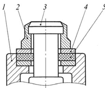
Рис. 8 – Демпфирующее устройство в кинематической цепочке подвижной системы ЭМП клапана: 1 – ползун; 2 – стопорная шайба; 3 – шток; 4 – шайба; 5 – пружинный элемент с малой жесткостью
