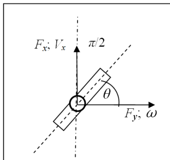
Рис. 2 – Геометрическая модель ДКР
