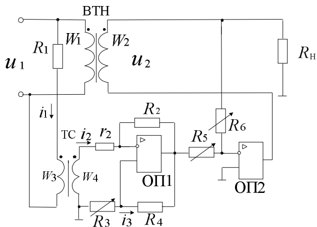
Рис. 2 - Схема компенсації похибки за допомогою ТС
