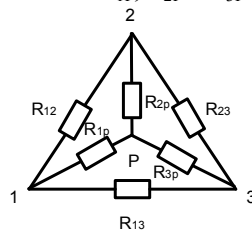
Рис. 4 - Преобразование треугольника в звезду
