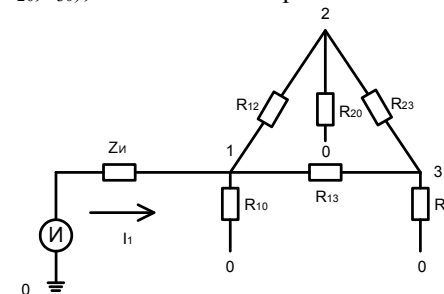
Рис. 2 - Использование элемента 1 как заземлителя для внешнего источника И(E, Z_{вн})
