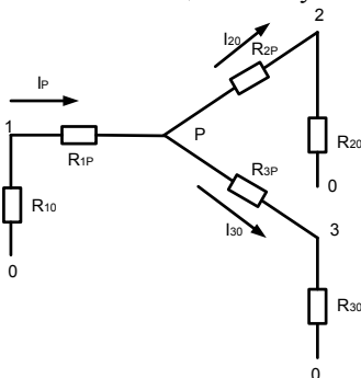
Рис. 5 - Схема замещения
