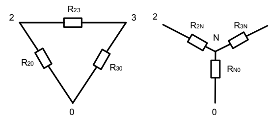
Рис. 3 - Преобразование треугольника в звезду
