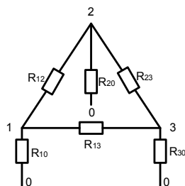
Рис. 1 - Схема замещения для трех взаимодействующих ( R_{12}, R_{23}, R_{13} ) элементов заземления ( R_{10}, R_{20}, R_{30} )
