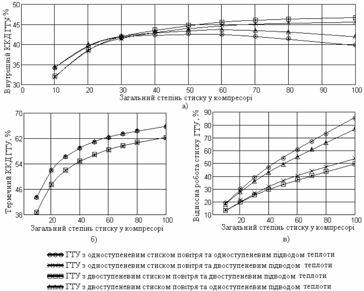
Рис. 6. Результати досліджень ускладнення циклу ГТУ відкритого типу на його параметри: температура газу на вході у ГТВДТ 1500 °С; степінь стиску у КНТ = 1,2; степінь розширення газу у ГТВДТ = 3
