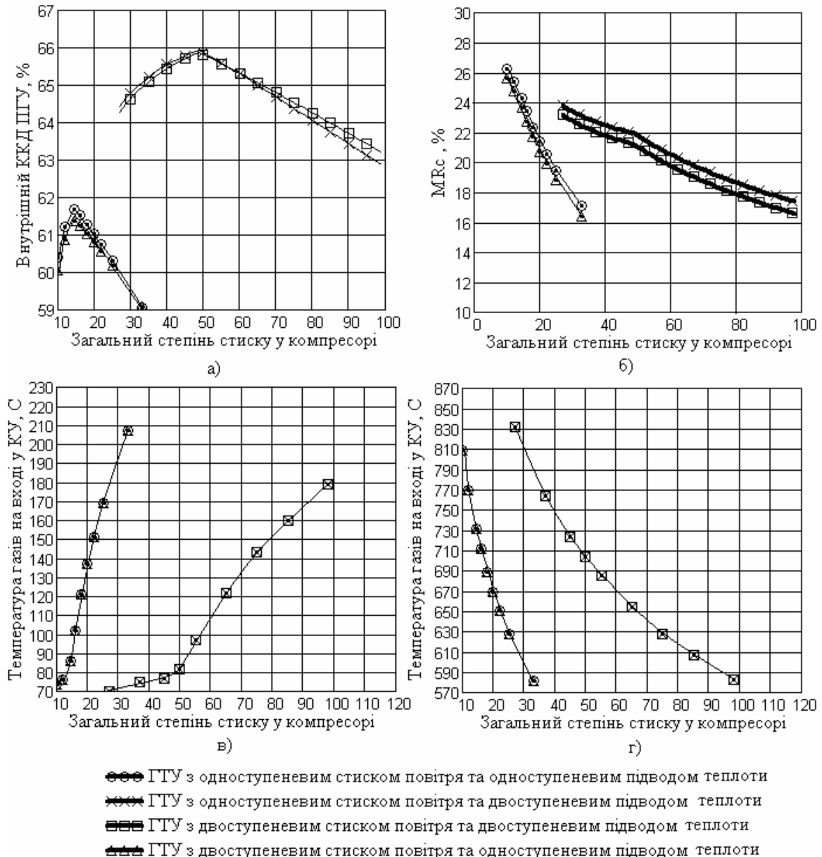
Рис. 7. Результати досліджень ускладнення циклу ПГУ на його параметри; температура газу на вході у ГТБТ 1500 °С; ступінь стиску у КНТ = 1,2; ступінь розширення газу у ГТБТ = 3
