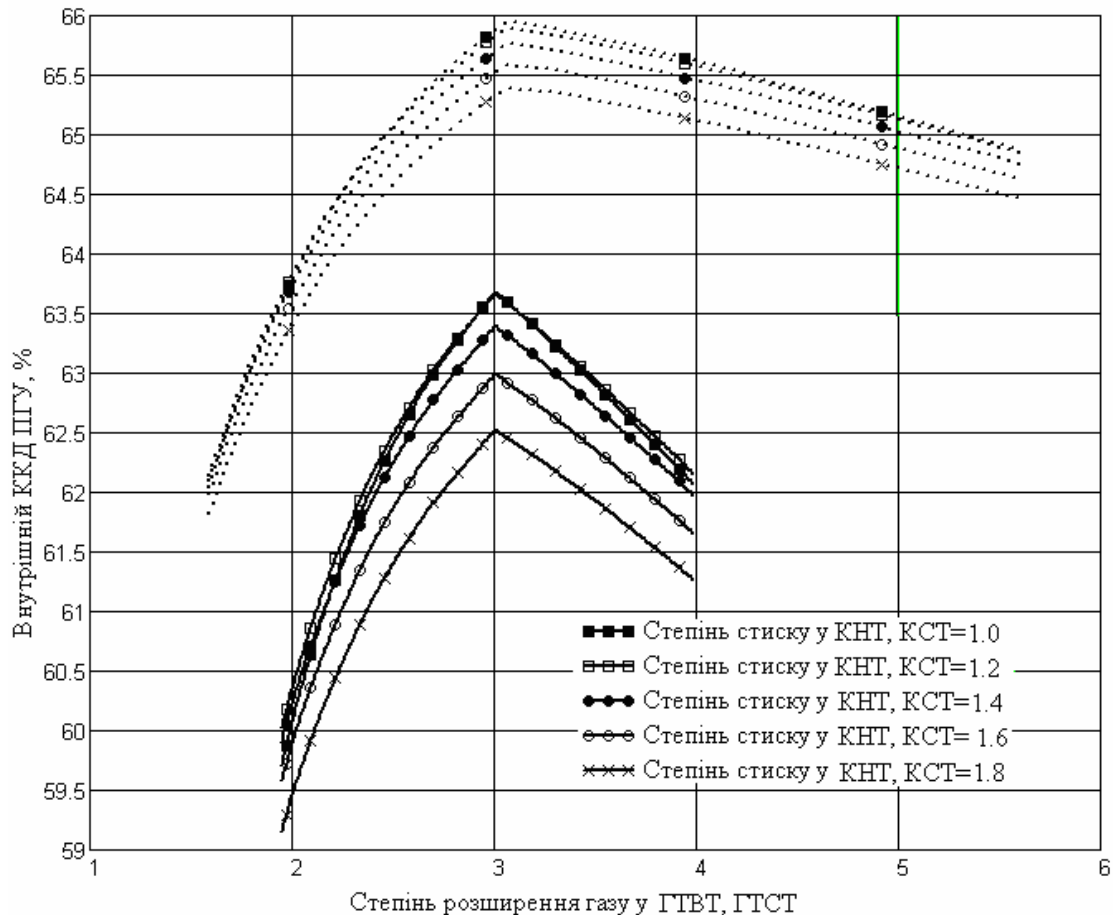
Рис. 9. Вплив степеня розширення газу у ГТВТ (при максимальній температурі газів у ГТУ 1500 °C) – штрихові лінії, та степеня розширення газу у ГТВТ та ГТСТ (при максимальній температурі газів у ГТУ 1200 °C) – суцільні лінії, на внутрішній ККД ПГУ КУ при загальному степені стиску повітря \pi_K = 50
