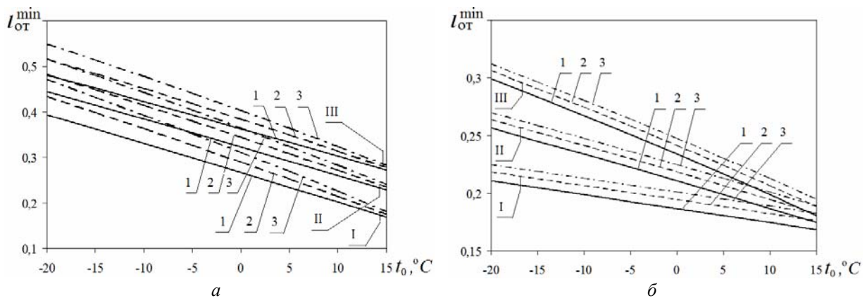
Рис. 5 – Зависимость минимальных удельных затрат внешней энергии на отопление от температуры окружающей среды: а – воздух: I, II, III – A = 0, 0,1, 0,5 ; 1 ( t - t_T^P = 30 \text{ }^\circ\text{C} ; 2 – 40 \text{ }^\circ\text{C} ; 3 – 50 \text{ }^\circ\text{C} ); б – грунт: I, II, III – t_T^P = 30; 40; 50 \text{ }^\circ\text{C} ( l - A = 0,005; 2 - 0,015; 3 - 0,027 )
