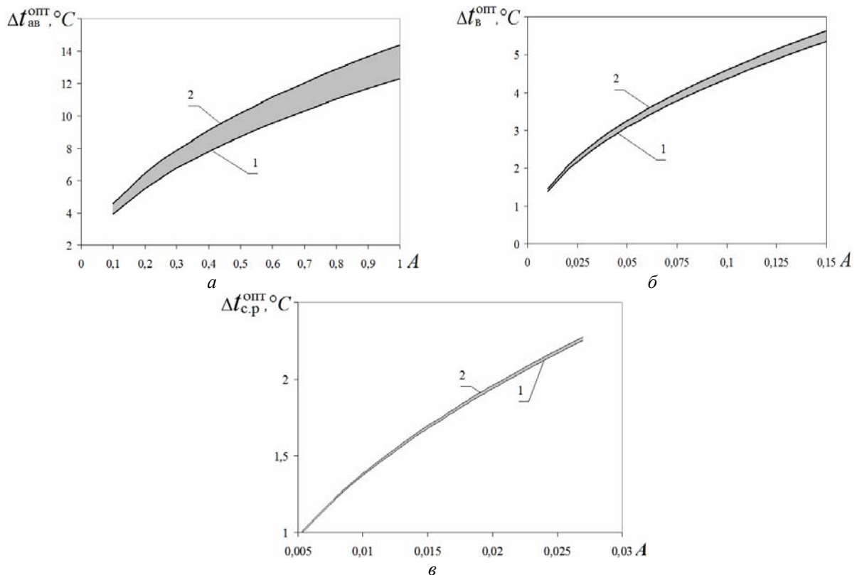
Рис. 2 – Зависимость оптимальной степени охлаждения среды в испарителе от комплекса заданных величин A : а – воздух: 1, 2 – для температуры атмосферного воздуха на входе в испаритель t_0 = -20\text{ }^\circ\text{C} и 15\text{ }^\circ\text{C} ; б – вода: 1, 2 – для температуры воды t_{в}^{вх} = 4\text{ }^\circ\text{C} и 20\text{ }^\circ\text{C} ; в – грунт: 1, 2 – температура соляного раствора t_{с.р.}^{вх} = 2\text{ }^\circ\text{C} и 5\text{ }^\circ\text{C}
