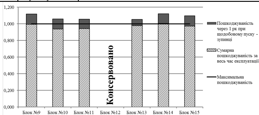
Рис. 7 – Діаграма прогнозованої пошкоджуваності блоків Луганської ТЕС (котел)
