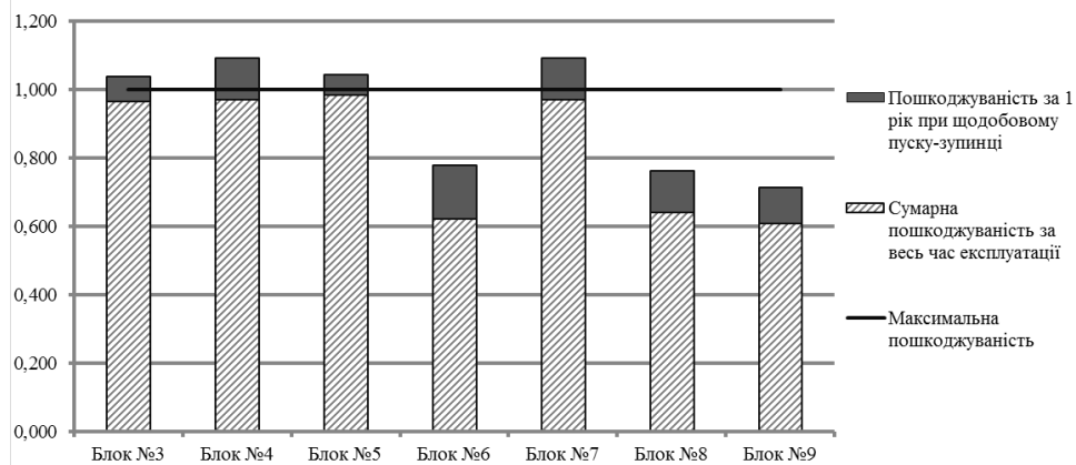
Рис. 1 – Діаграма прогнозованої пошкоджуваності блоків Кураховської ТЕС (турбіна)
