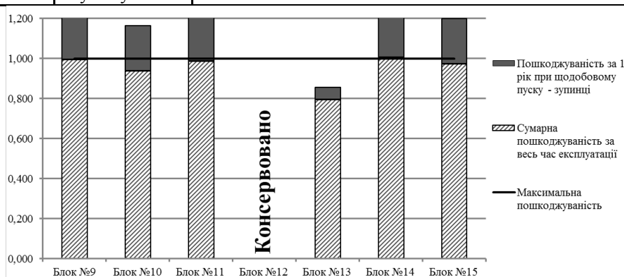
Рис. 5 – Діаграма прогнозованої пошкоджуваності блоків Луганської ТЕС (турбіна)
