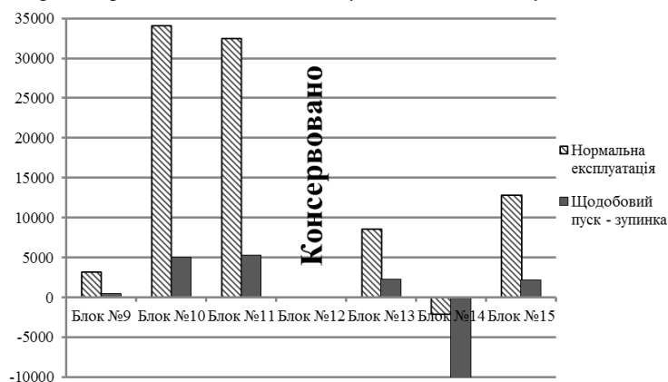
Рис. 8 – Прогнозований залишковий ресурс блоків Луганської ТЕС (котел)
