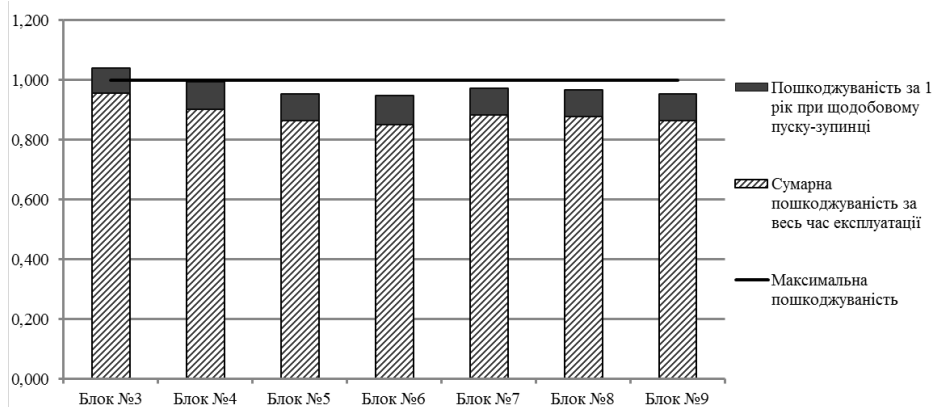
Рис. 3 – Діаграма прогнозованої пошкоджувальності блоків Кураховської ТЕС (котел)
