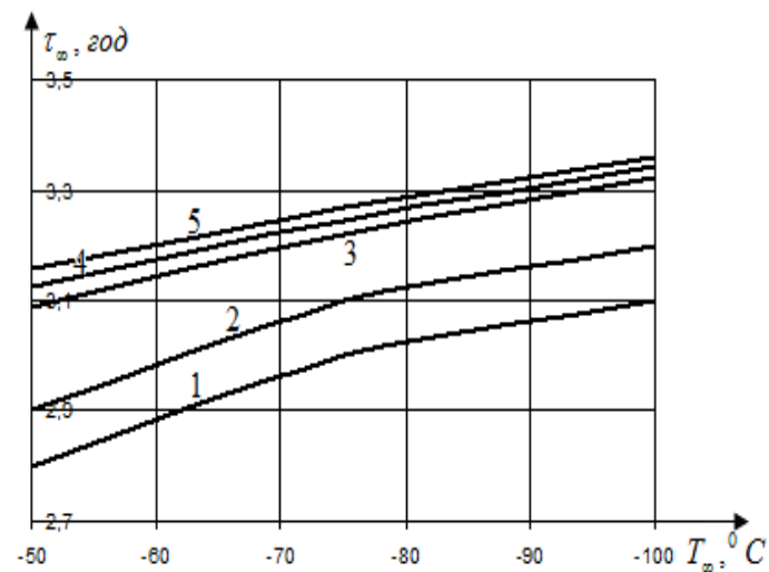
Рис. 5 – Інтервал часу, необхідний для просування фронту фазового перетворення всередину стінки фільтру: 1 – T_0 = 5 °C; 2 – T_0 = 10 °C; 3 – T_0 = 15 °C; 4 – T_0 = 20 °C; 5 – T_0 = 25 °C
