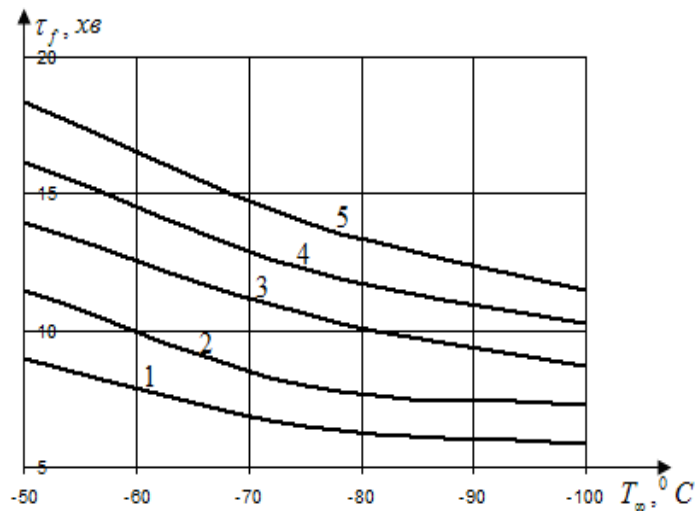
Рис. 4 – Інтервал часу, необхідний для просування фронту фазового перетворення всередину стінки фільтру: 1 – T_0 = 5 °C; 2 – T_0 = 10 °C; 3 – T_0 = 15 °C; 4 – T_0 = 20 °C; 5 – T_0 = 25 °C
