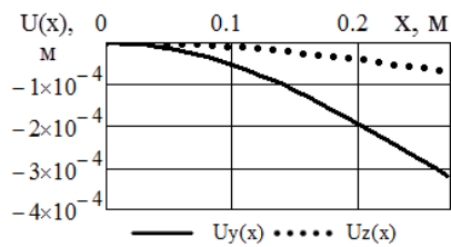
Рис. 2 – Амплитуды вынужденных колебаний
