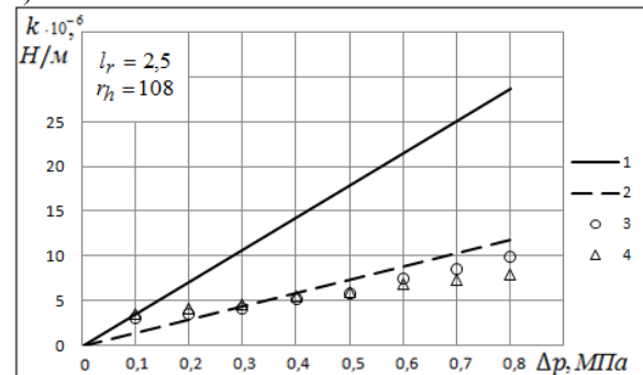
Рис. 7 – Теоретические и экспериментальные зависимости коэффициента радиальной жёсткости гидростатической силы
