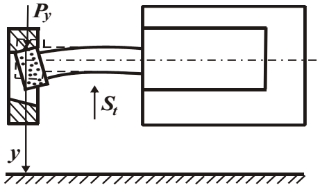
Рис. 1 – Розрахункова схема параметрів внутрішнього шліфування.
