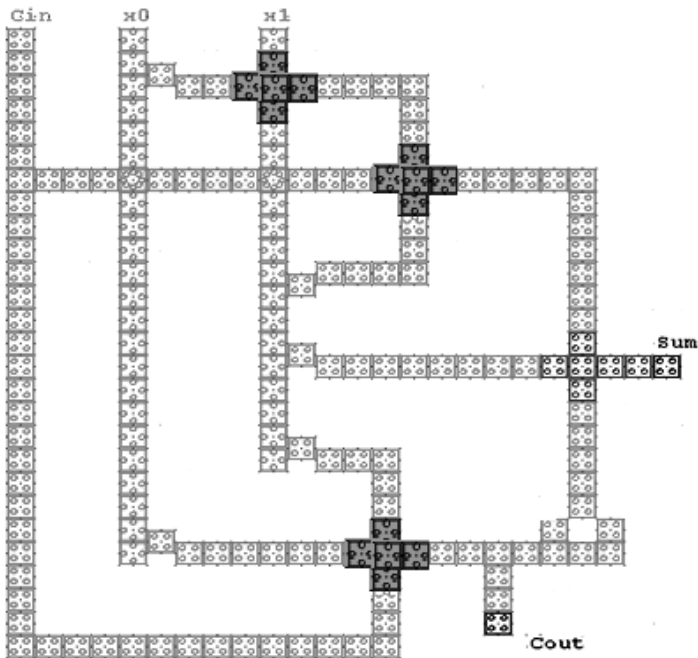
Рис. 5 – Наносхема суматора на квантових коміркових автоматах.
