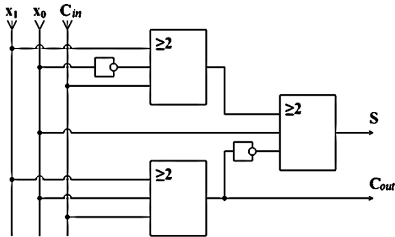
Рис. 4 – Схема однорозрядного суматора на мажоритарних елементах.
