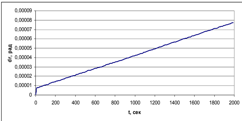
Рис. 2 – Оцінка похибки дрейфу, отримана на еталонній моделі регулярної прецесії при початкових умовах (17): а – для алгоритму першого порядку; б – для обчислень по двосітковій схемі
