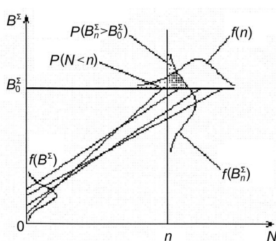
Рис. 2 – Модель підсумовування пошкоджуваностей за r = 1 .
