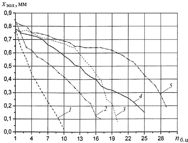
Рис. 4 – Залежність ходу золотника від кількості блок-циклів напрацювання (1 блок-цикл дорівнює 20000 циклів) для п'яти клапанів: 1, 2, 3, 4, 5 – номери клапанів.
