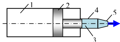
Рис. 2 – Импульсный водомет: 1 – сжатый газ, 2 – поршень, 3 – вода, 4 – ствол, 5 – сопло.
