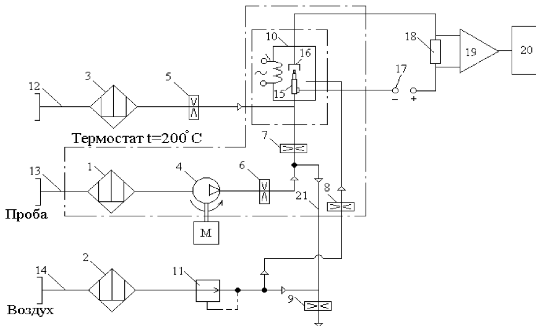
Рис. 1 – Структурная схема ПИД: 1,2,3 - фільтри, 4-компрессор, 5-9 - дросель, 10 – корпус ионизационной камеры, 11- регулятор давления, 12- генератор водорода, 13 – газопровод для пробы, 14 газопровод воздуха, 15 – горелка, 16 – электрод-коллектор, 17 – источник питания, 18 – нагрузочное сопротивление, 19 - электрометрический усилитель, 20- выходной прибор
