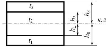
Рис. 2. Схема тришарового стержня, який оброблений алмазним вигладжуванням.
