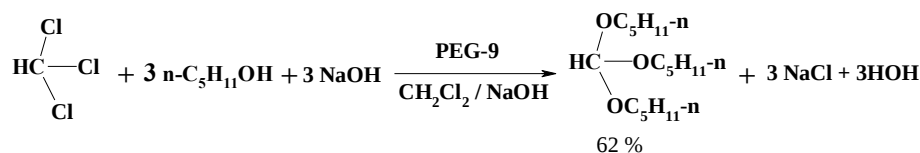
ис. 4 - Схема синтеза три- n -пентилортоформиата в гетерофазной системе при катализе ПЭГ-9
