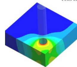
Рис. 25 – Распределения полных перемещений в нижней базовой плите штампа при натяге 0,1 мм (задача 2.1)
