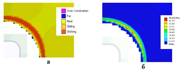
Рис. 11 – Результати дослідження НДС елементів штамп в сопряженні подштамповою плити преса и базовою плити штамп (задача 1): а – розподілення контактних зон; б – розподілення контактних давлень
