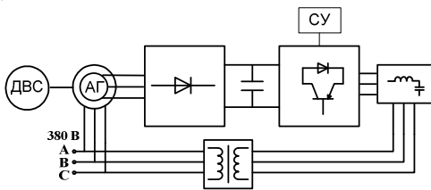
Рис. 1 – Схема испытательного стенда на базе АГ и АПН.
