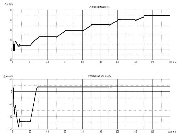
Рис. 11 – График передаваемой активной и реактивной мощности инвертором.
