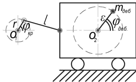
Рис. 1 – Кинематическая схема
