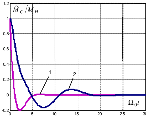
Рис. 5. Графіки похибки оцінювання статичної складової електромагнітного моменту АД за допомогою спрощених спостерігачів, що застосовують корекцію за швидкістю (криві 1) та за активною складовою струму статора (криві 2), при накладанні номінального навантаження на усталеній швидкості.
