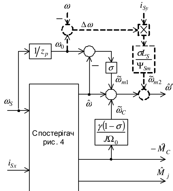
Рис. 6. Спостерігач з корекцією за активною складовою вектора струму статора з компенсацією усталеної похибки оцінювання.
