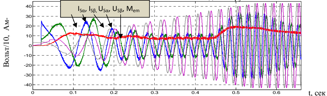
Рис. 3 Компоненти векторів напруги завдання, струму статора та електромагнітний момент АД.
