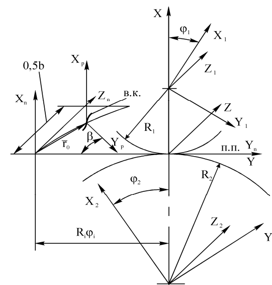
Рисунок – Системи координат у верстатному зачепленні
