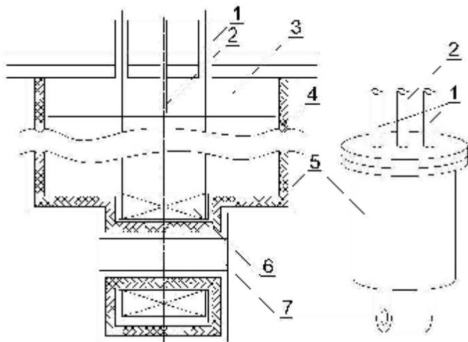
Рис. 9. Схематический вид криосистемы соленоида: 1 – тоководы соленоида, 2 – переливочка для заливки жидкого гелия, 3 – объем с жидким гелием или область размещения криогенератора, 4 – слоистая вакуумная теплоизоляция или азотный экран, 5 – корпус дьюара или криогенератора, 6 – соленоид, 7 – отверстие для ввода пучка
