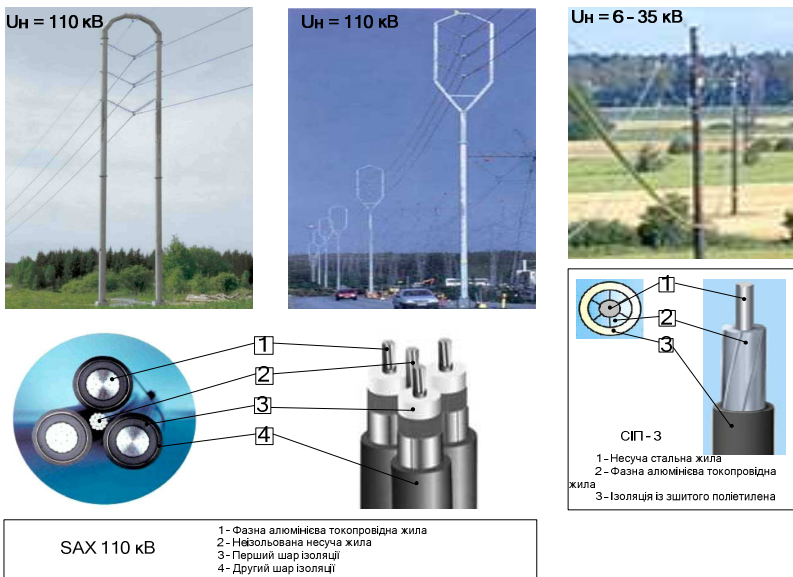
Рис. 2. ВЛ напругою 6-35 кВ і 110 кВ, виконані самонесущим кабелем повітряної підвіски. Конструкція кабелів для ВЛ даних класів напруги
