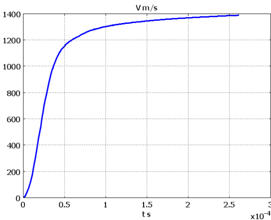
Рис. 2 – Временная зависимость скорости системы.
