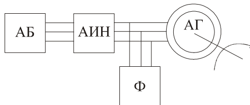
Рис. 2 – Схема генерирования тока АГ с вентильным возбуждением
