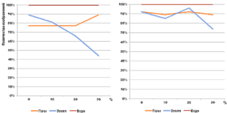
Рис. 3. Залежність якості навчання від навчальної вибірки для текстур 64x64 з нормальною навчальною вибіркою та зашумленою навчальною вибіркою (рівномірне зашумлення)
