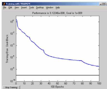
Рис. 1. Графічний інтерфейс системи розпізнавання. Навчання нейронної мережі
