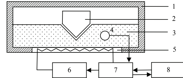
1 – корпус; 2 – объект; 3 – нагреватель; 4 – датчик температуры; 5 – элемент Пельтье; 6 – источник питания; 7 – блок управления; 8 – внешнее устройство (ПЭВМ)
