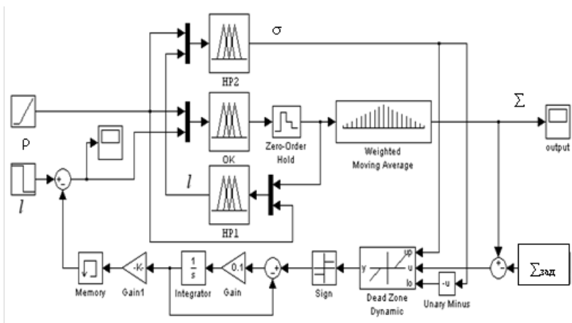
Рисунок 2 – Структура моделі адаптивної системи керування з HP1, HP2
