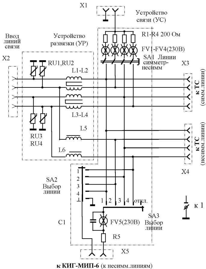
Рисунок 4 – Схема электрическая принципиальная устройства связи-развязки УСР-МИП (НЭЛС)
