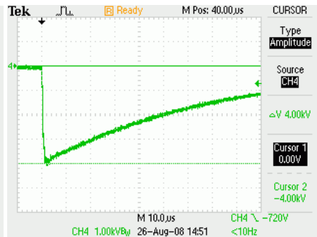
Рисунок 10 – Импульс напряжения отрицательной полярности A = -4 кВ на ненагруженном выходе испытательного генератора
