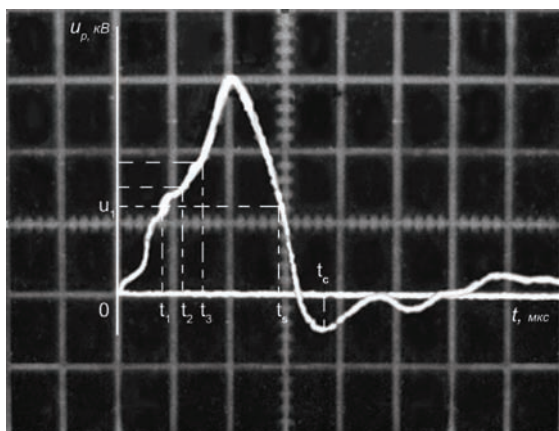
Типовая форма ВСХ импульсного напряжения u_p(t) на разрядниках замыкателях нагрузки генератора ГБИТМ
