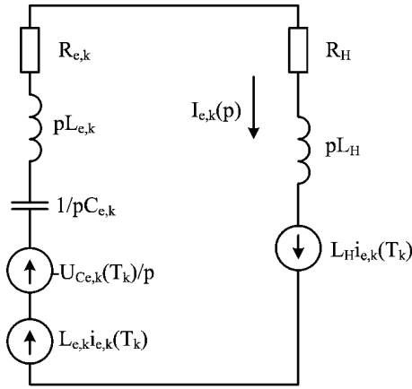
Рисунок 2 – Эквивалентная послекоммутационная схема:
