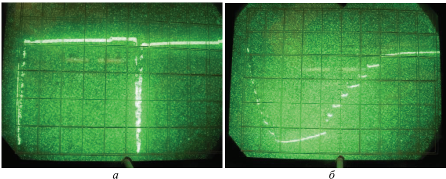
Рисунок 3 – Импульсы напряжения на емкостно-омической нагрузке (в виде реактора с коронным разрядом) высоковольтного импульсного трансформатора без обострения фронта импульсов (1 В/дел, k_d = 5260 ): а – 200 мкс/дел, б – 5 мкс/дел
