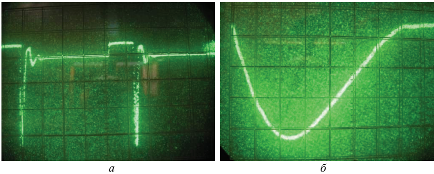
Рисунок 2 – Импульсы напряжения на резистивной нагрузке высоковольтного импульсного трансформатора (1 В/дел, k_d = 5260 ): а – 200 мкс/дел, б – 5 мкс/дел
