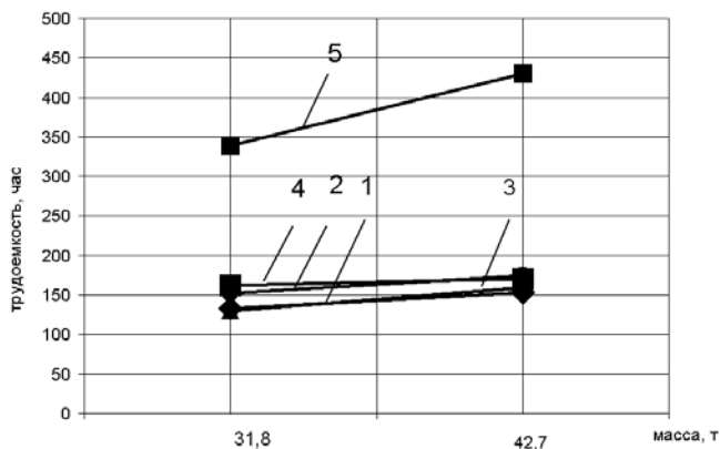
Рис. 9. Характер изменения трудоемкости (относительно общей трудоемкости) при изготовлении нового составного шпинделя): – левой головки (меньшей) (1); - правой головки (большей) (2); – вала шпинделя (3); – при сборке изделия (4); - при окончательной механической обработке изделия (5) в зависимости от изменения типоразмера изделия (в частности, массы)
