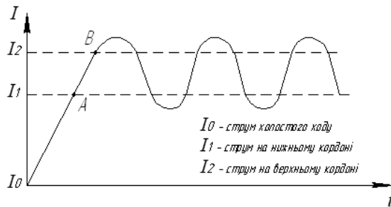
Рисунок 2 – Струм електромотору
