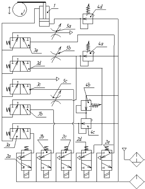
Рисунок 1 – Пневматична схема керування пневмоциліндром шліфувальної бабки (прототип)
