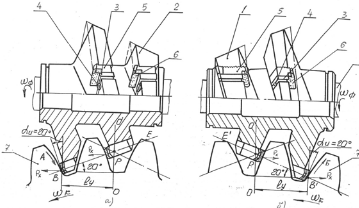
Рис.1 – Двухкорпусная фреза одностороннего резания. а – правый корпус; б – левый корпус.
