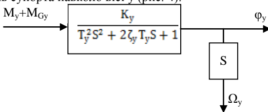
Рисунок 4 – Структурна математична модель для визначення параметрів поперечно-кутових коливань супорта навколо вісі у.
