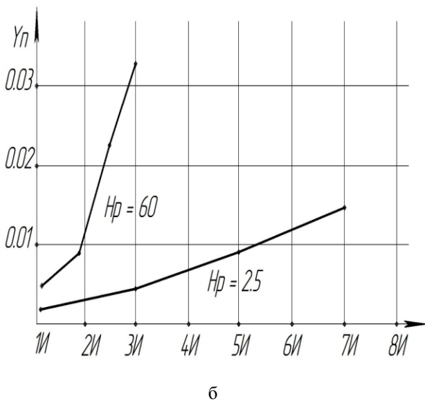
Рис. 10 – Величина линейного смещения вершины реза: а – традиционная методика регламентации качества поверхности, б – регламентация при помощи КП; ( H_r – высота сглаживания макроотклонений, мкм)
