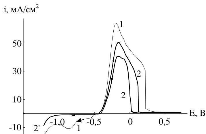
Рис. 3. Прямий(1, 2) та зворотний(1',2') хід поляризаційних кривих сталі у 0,5М нітратному розчині без добавок (1,1') та з добавкою 3 г/дм 3 Na 2 MoO 4 (2, 2') при рН 1,7
