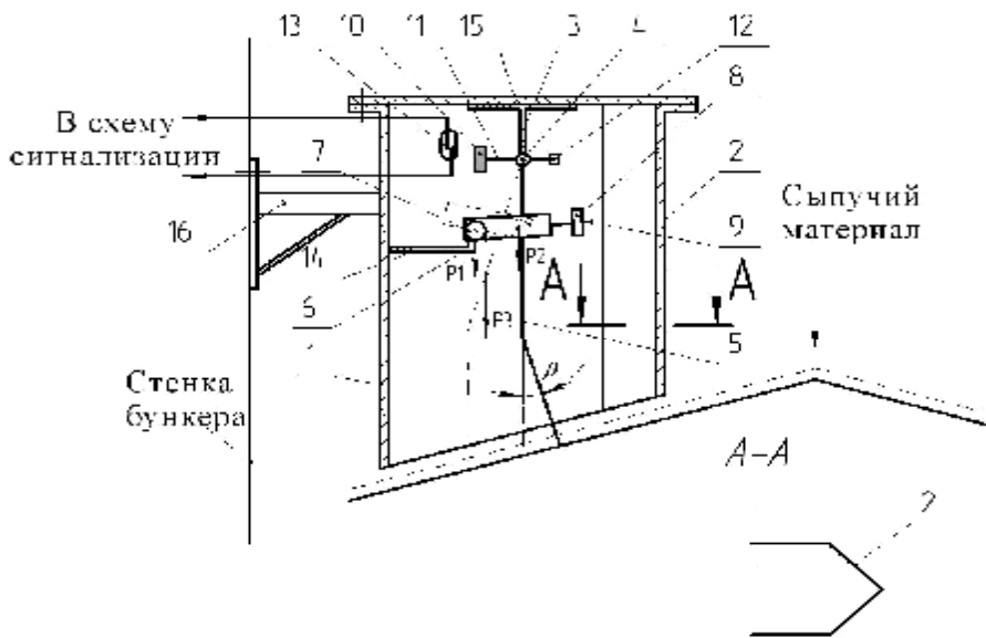
Рис. 1. Сигнализатор уровня
