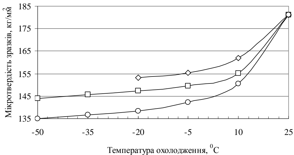
Рис. 2. Залежність мікротвердості вторинної вольфрамвмісної сировини від температури охолоджувальної суміші на основі \text{NaCl} (-), \text{MgCl}_2 ( \text{€} ) і \text{AlCl}_3 ( \text{™} ).
