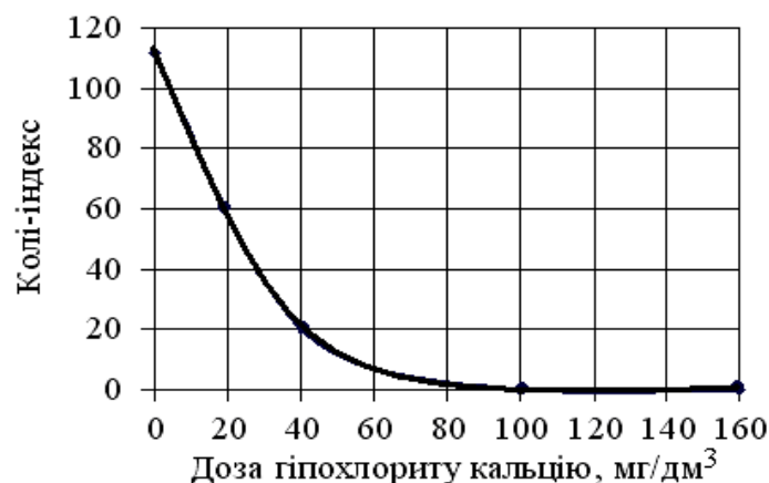
Рис. 2. Залежність колі-індексу очищеної води від дози гіпохлориту кальцію
