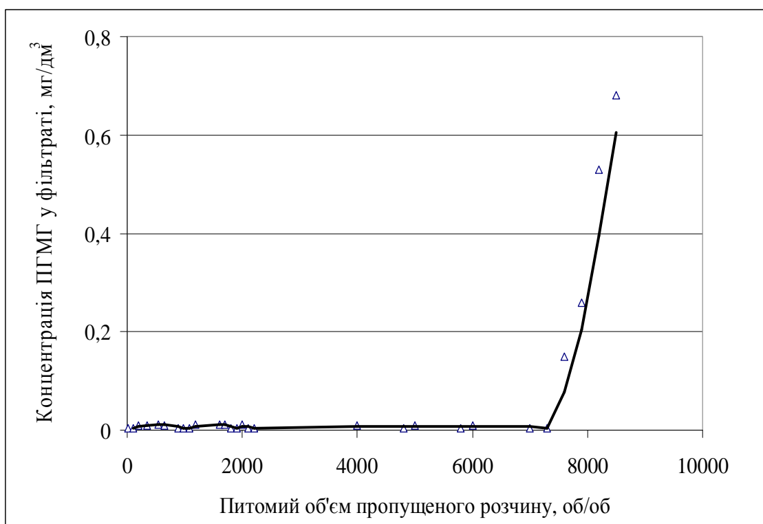
Рис. 1. Вихідна крива сорбції ПГМГ на іоніті № 1
