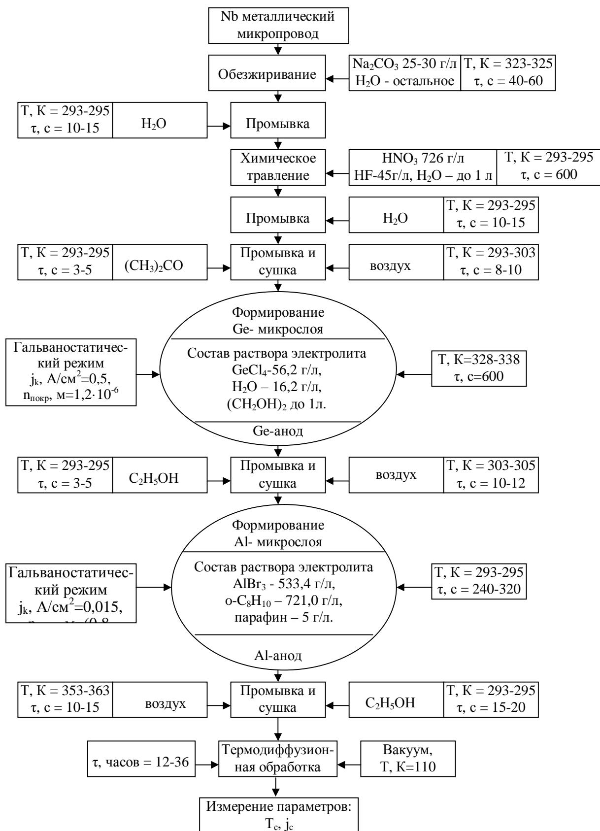
Рис. 2. Алгоритм проведения технологического процесса образования субмикроструктурированных полислоистых металлических структур типа Nb/Ge/Al и получения СП-фазы \text{Nb}_3\text{Ge}_x\text{Al}_{1-x}
