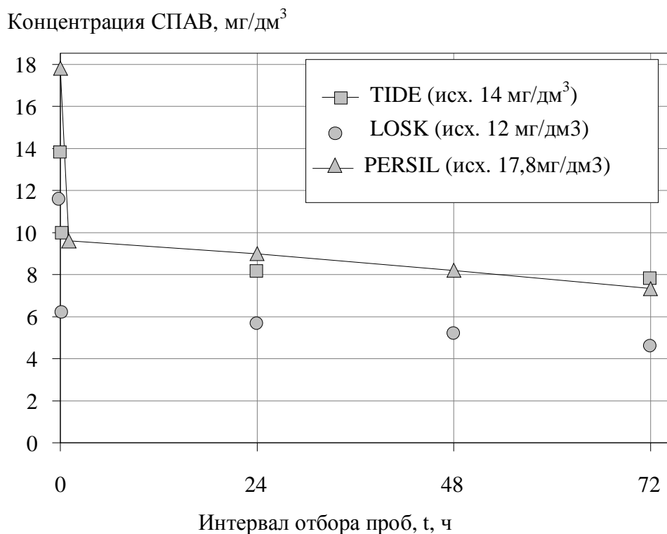
Рис. 1. Зависимость концентрации СПАВ от продолжительности обработки сточных вод в септике
