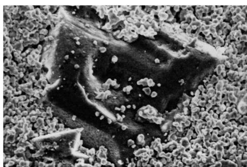
Рис. 2. Фрагмент рабочей поверхности диска с единичным зерном алмаза (×2000)
